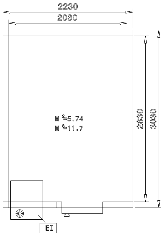
Zij aanzicht
